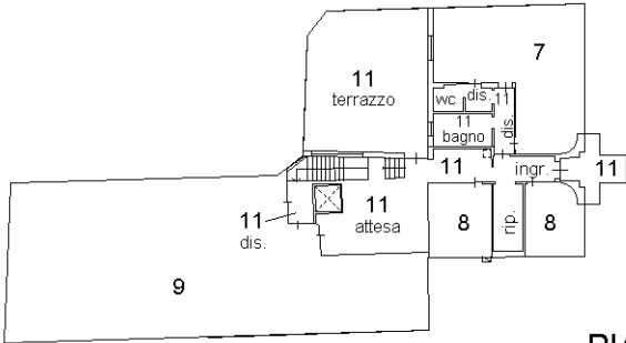
PIANO PRIMO
