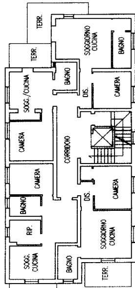
PIANTA PIANO SECONDO H = 2.80
