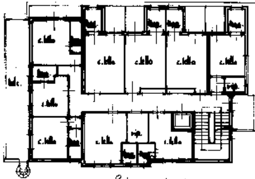
Piano primo piano - h. 200.
